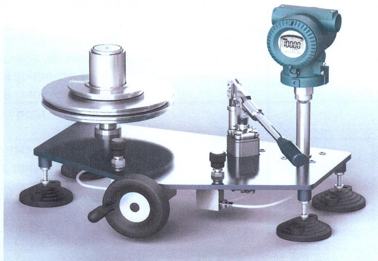
Рис. 2. Манометры газовые грузопоршневые МГП-2,5; МГП-10; МГП-100
