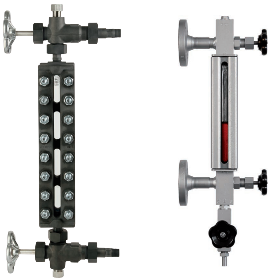
Стеклянный указатель уровня, модель LGG (примеры)
